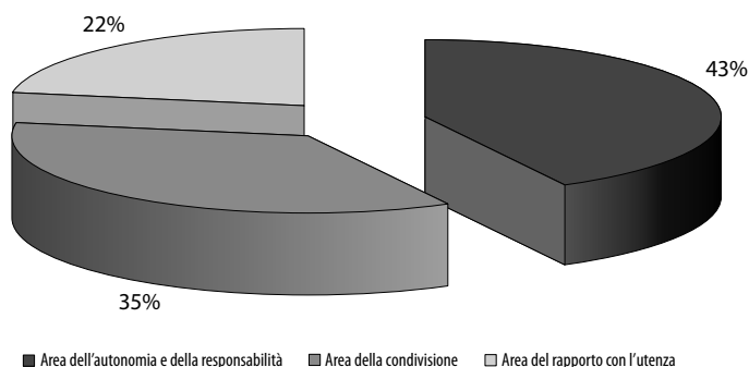
Figura 15. Indice sintetico
